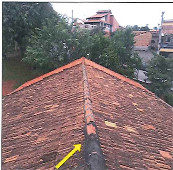
FOTO 03: VISTA DA CUMEEIRA NECESSITANDO DE REVISÃO. 21/03/2019 - 14:59
